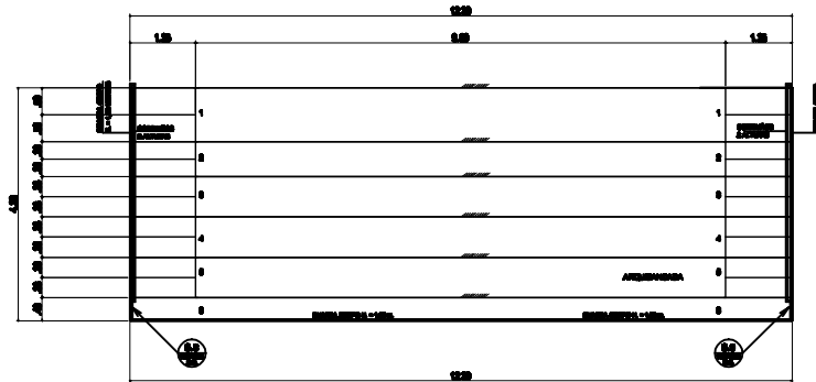
6 DETALHE ARQUIBANCADA (2 VEZES)
