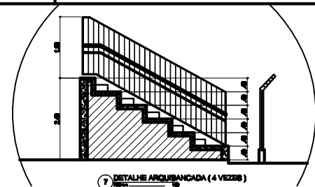
7 DETALHE ARQUIBANCADA (4 VEZES)
